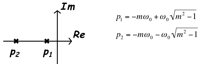
Fig. II.10 – Lieu des pôles pour m \gg 1 .
